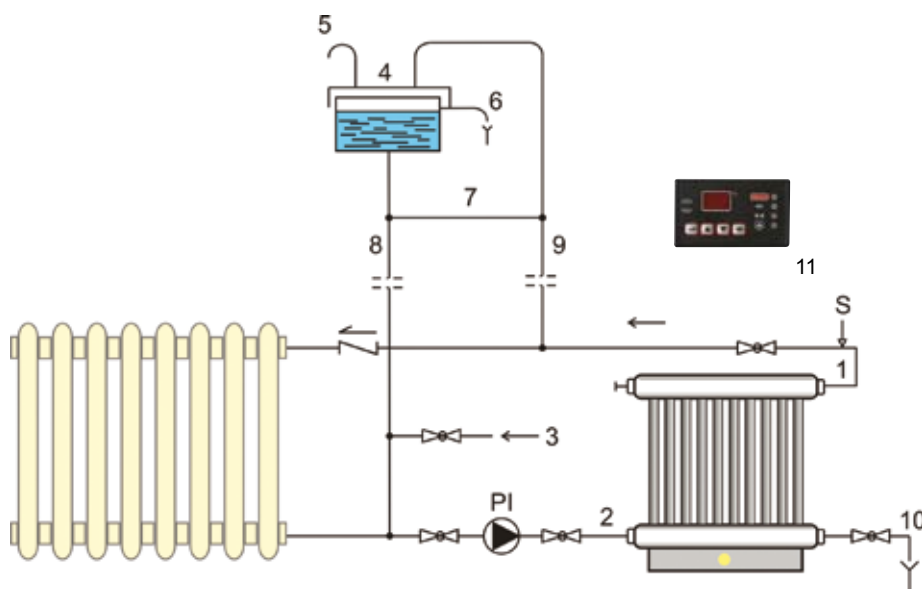
Schema indicativo di impianto a vaso aperto con scambiatore Indicative plan open vessel system for exchanger
